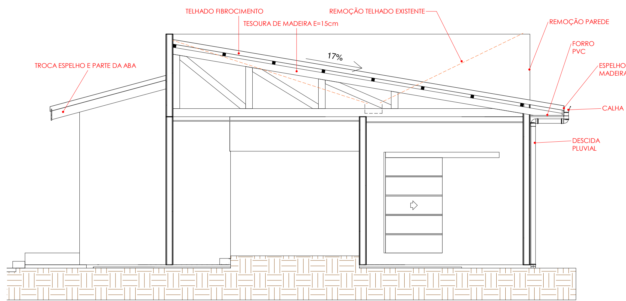
2 Corte A 1 : 50
