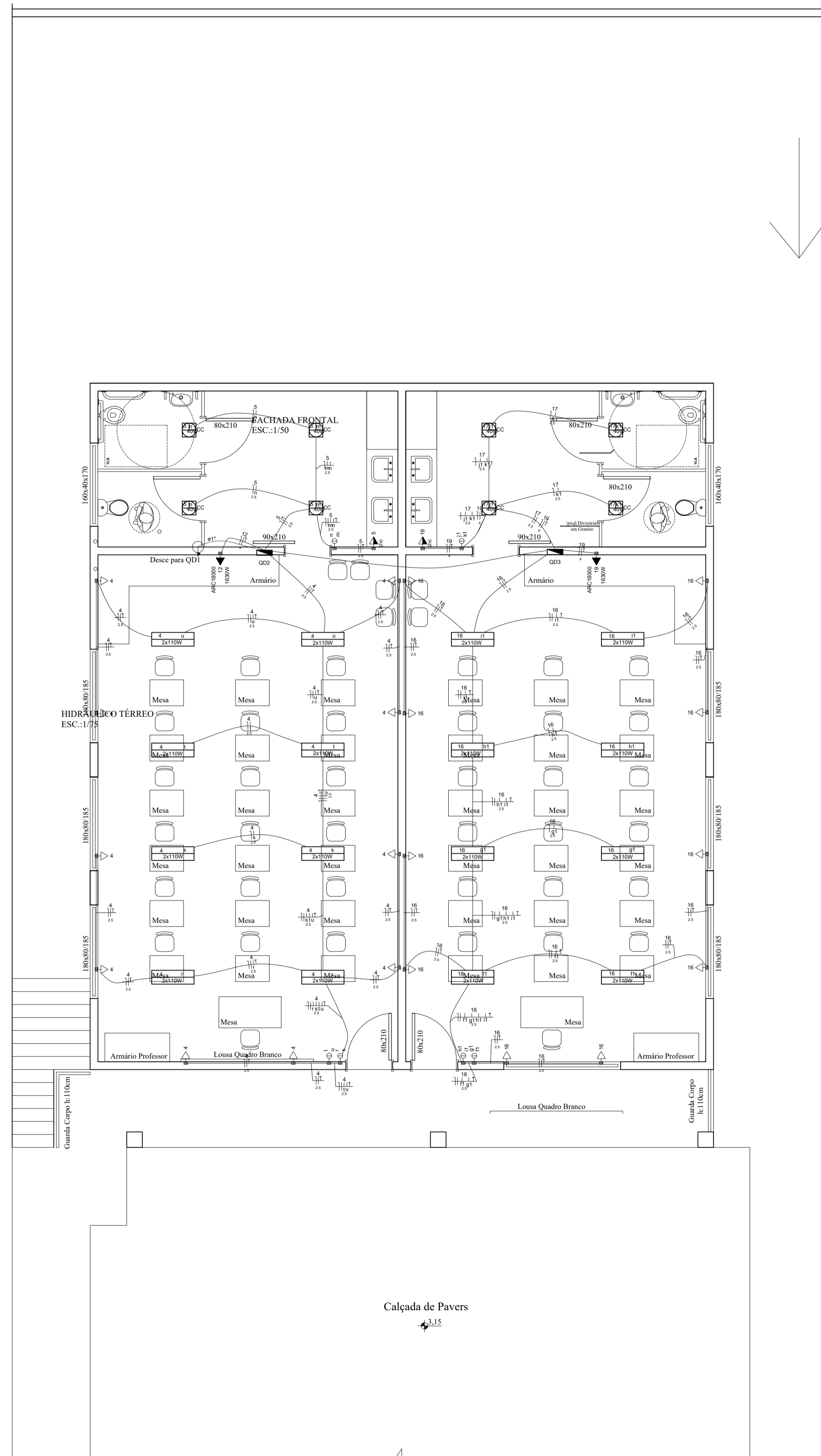
ELÉTRICO TÉRREO ESC.:1/75
