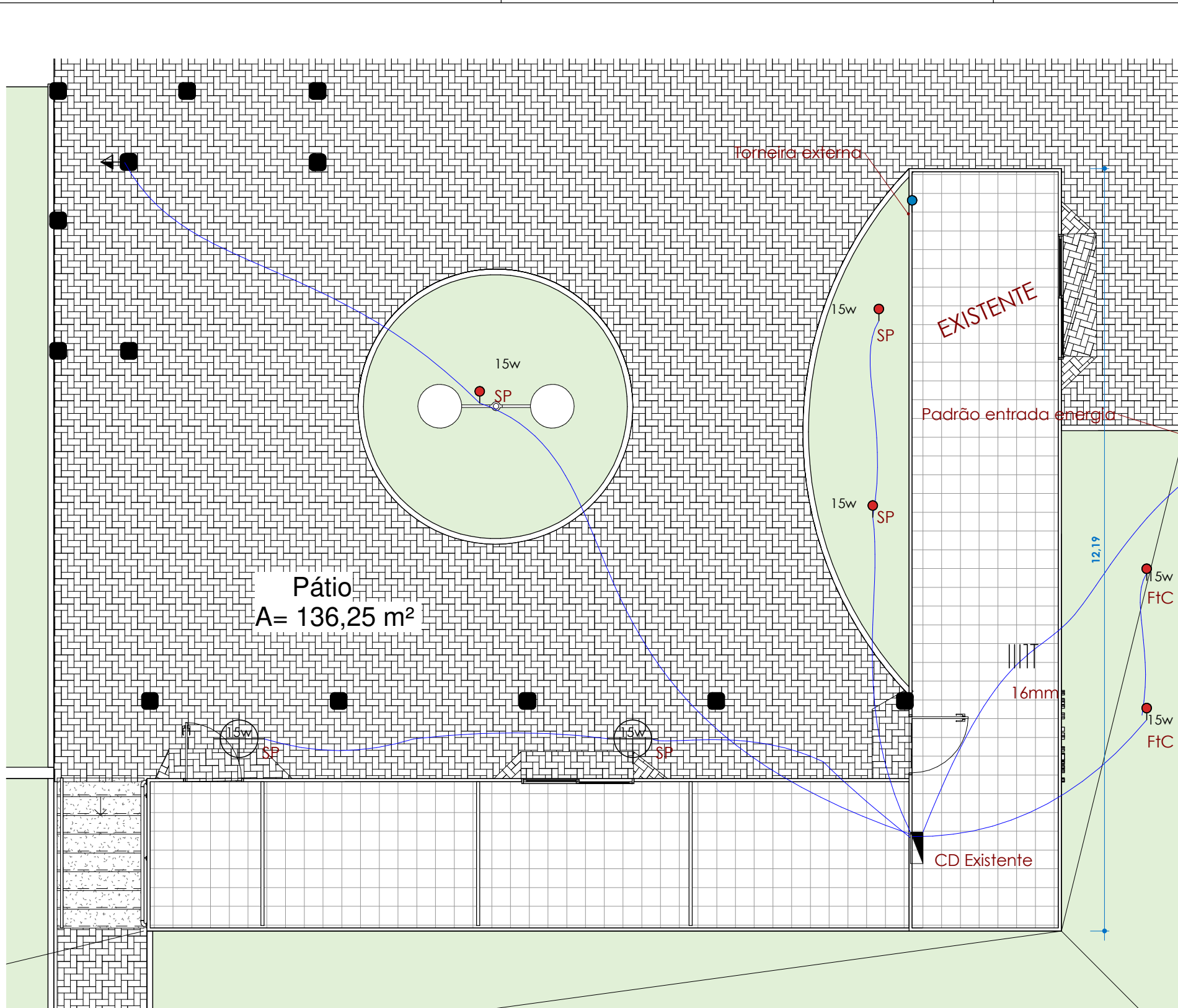
1 Terreo Elétrico 1 : 75
