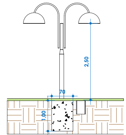
2 Det. Poste 1 : 75
