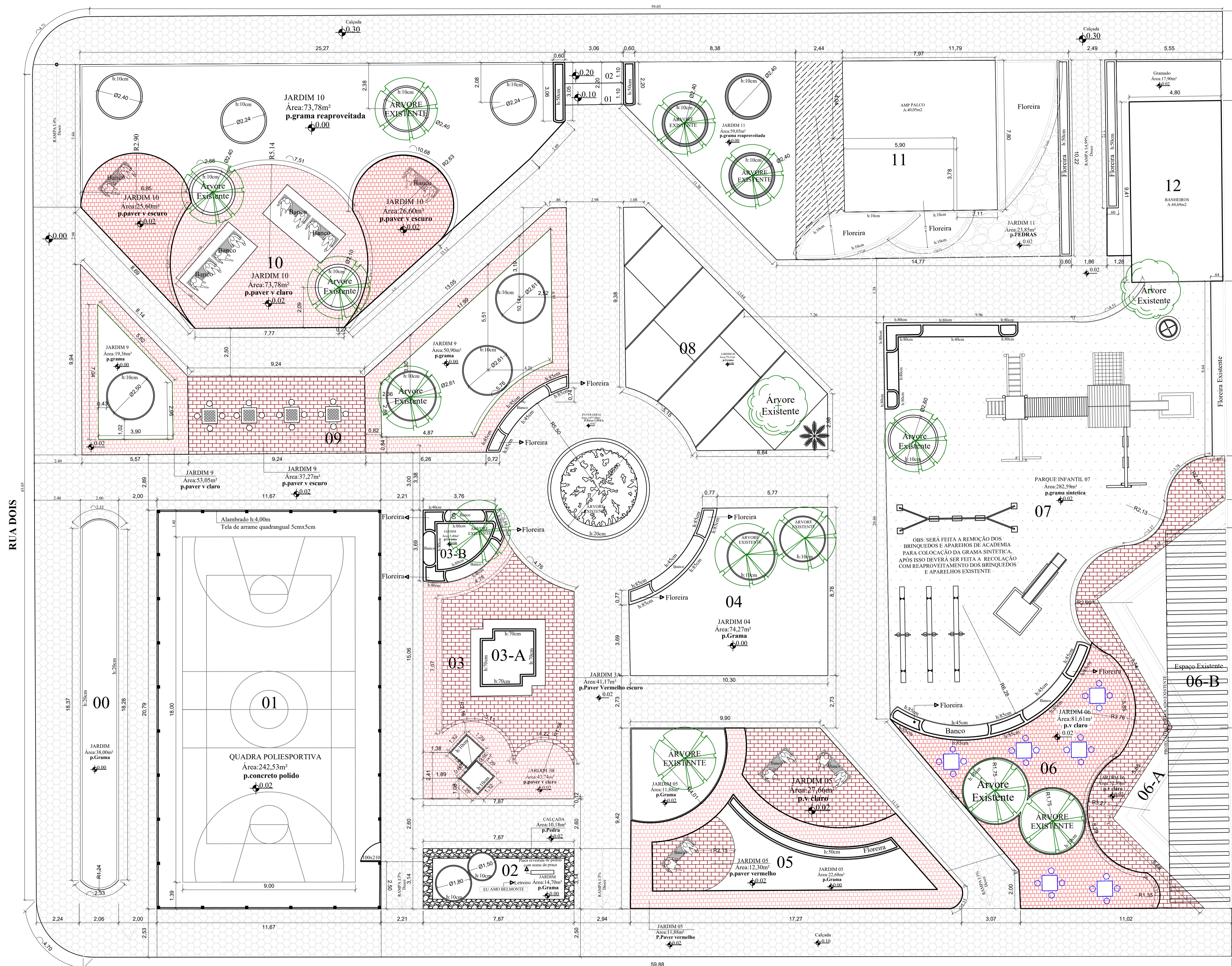
Planta Baixa Esc 1:50
