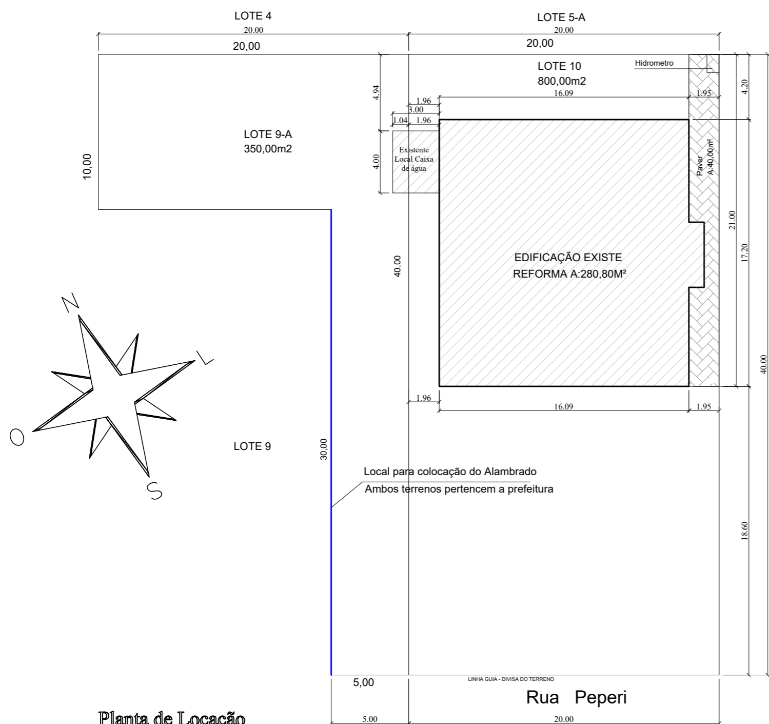
Planta de Locação Esc.: 1/250
