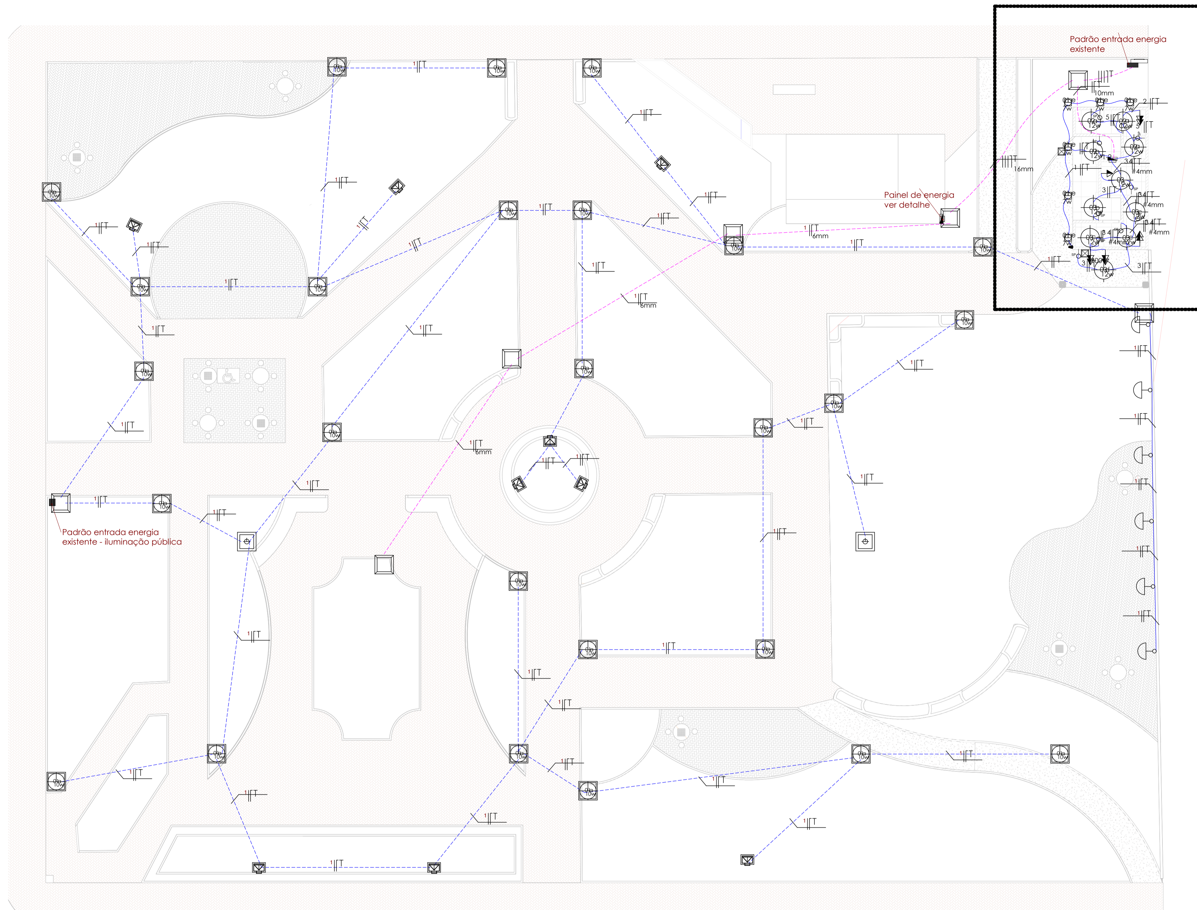
1 Distribuição Elétrica 1 : 125
