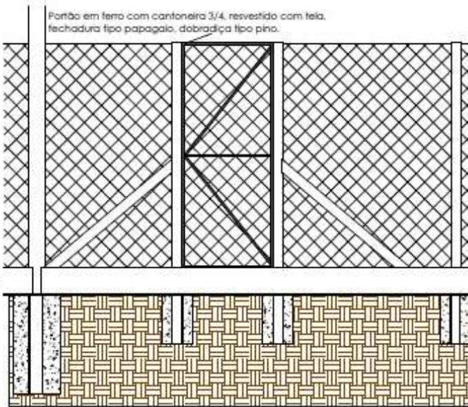
4 Detalhe Portão ferro 1:20
