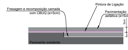
Detalhe Execução Remendo Superficial
