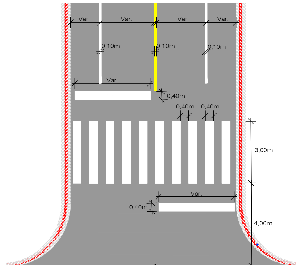
DETALHE SINALIZAÇÃO VIÁRIA S/ESCALA
