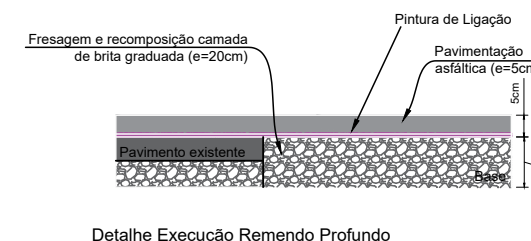
Detalhe Execução Remendo Profundo
