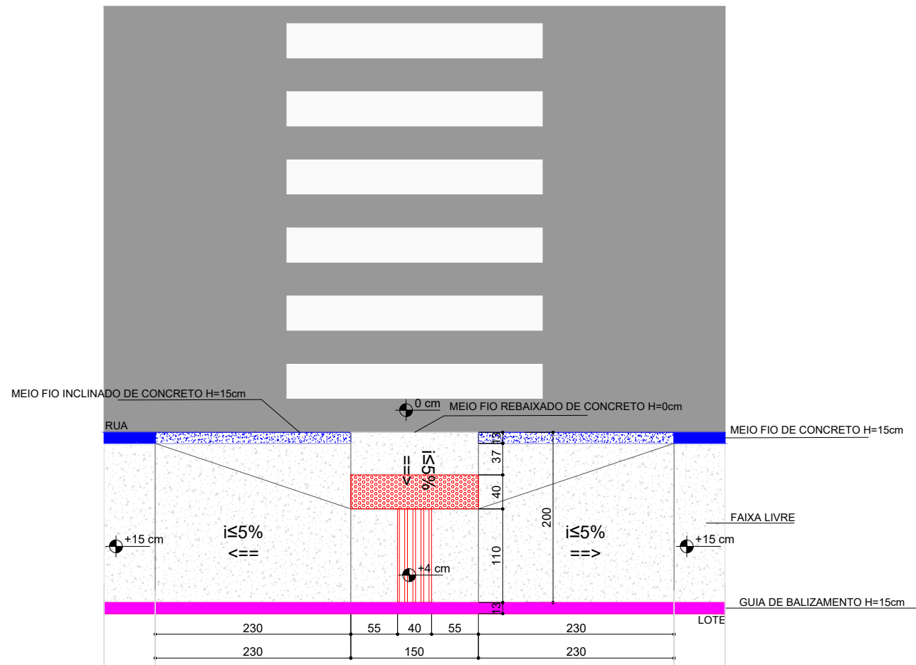
DETALHE RAMPA P.N.E S/ESCALA
